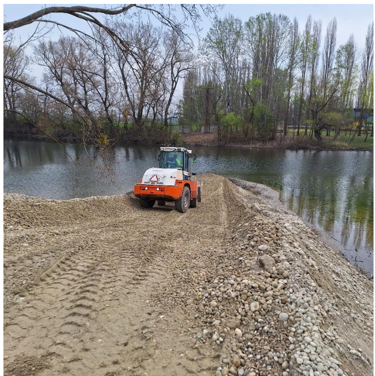
Úprava prístupovej komunikácie k ostrovu č. 1
