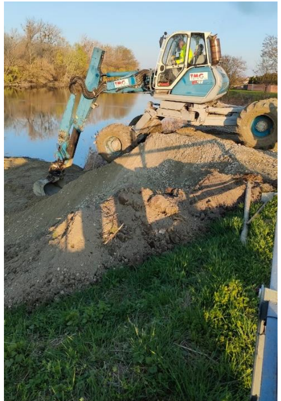
Svahovanie prístupovej rampy k štrkovej lavici č. 1
