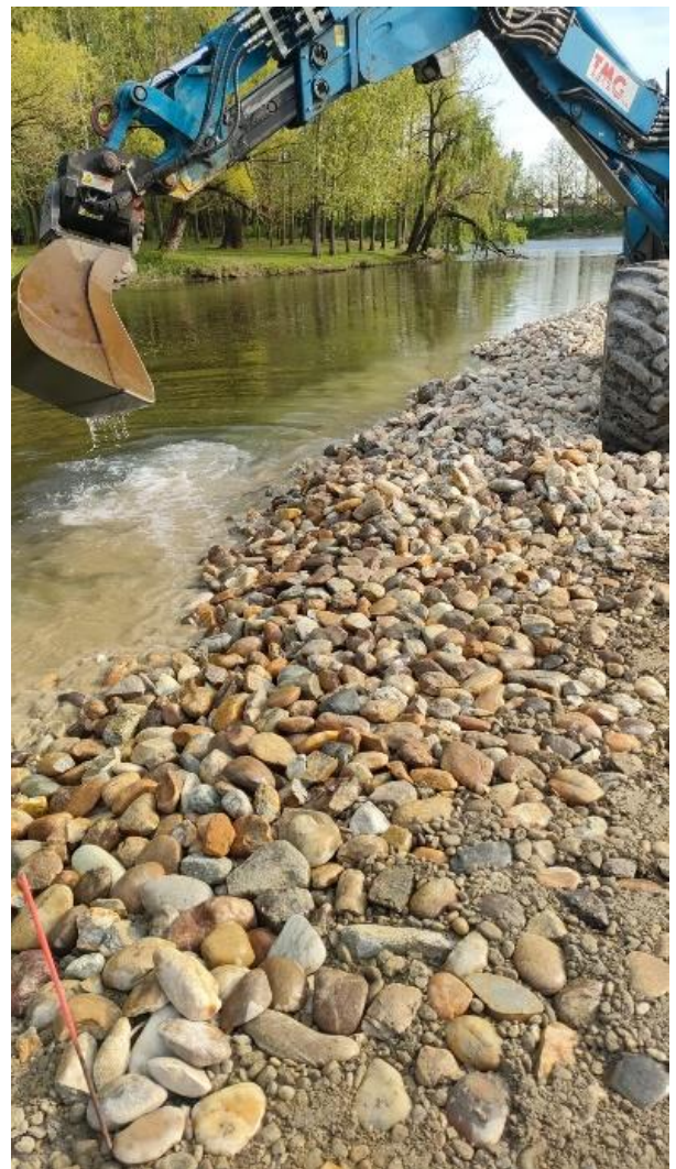
Opevnenie vonkajšieho svahu ostrova č. 1 hrubým riečnym kamenivom
