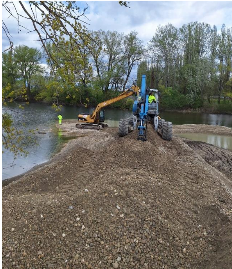
Nakladanie neufahnutého výkopku
