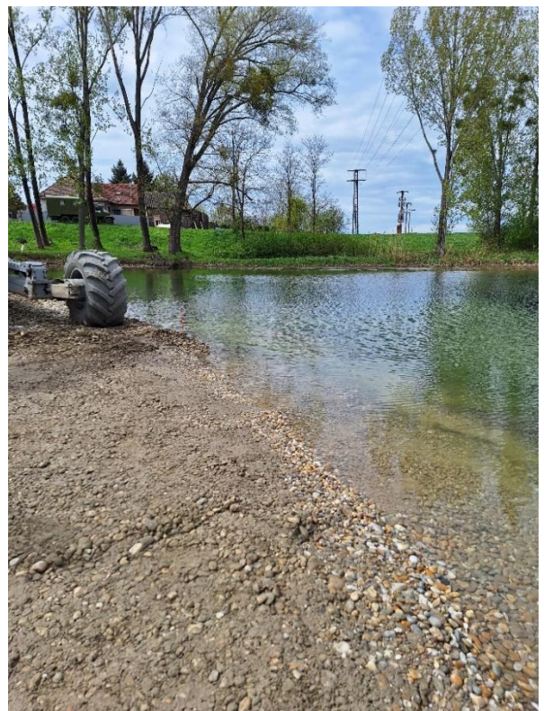
Svahovanie vonkajšieho obrysu ostrova č. 1
